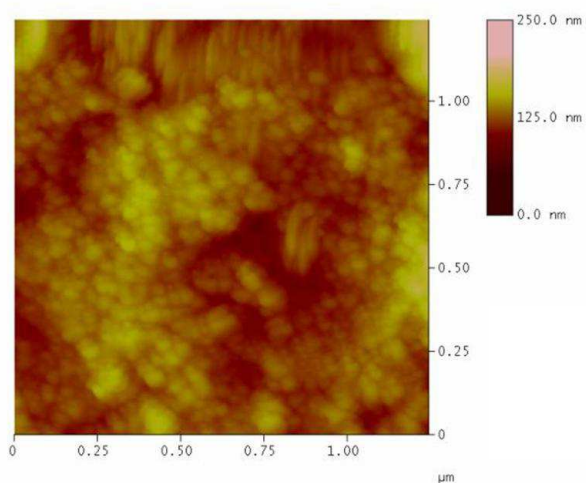
Slika 4 – AFM snimak površine nanotubularnog sloja TiO 2
