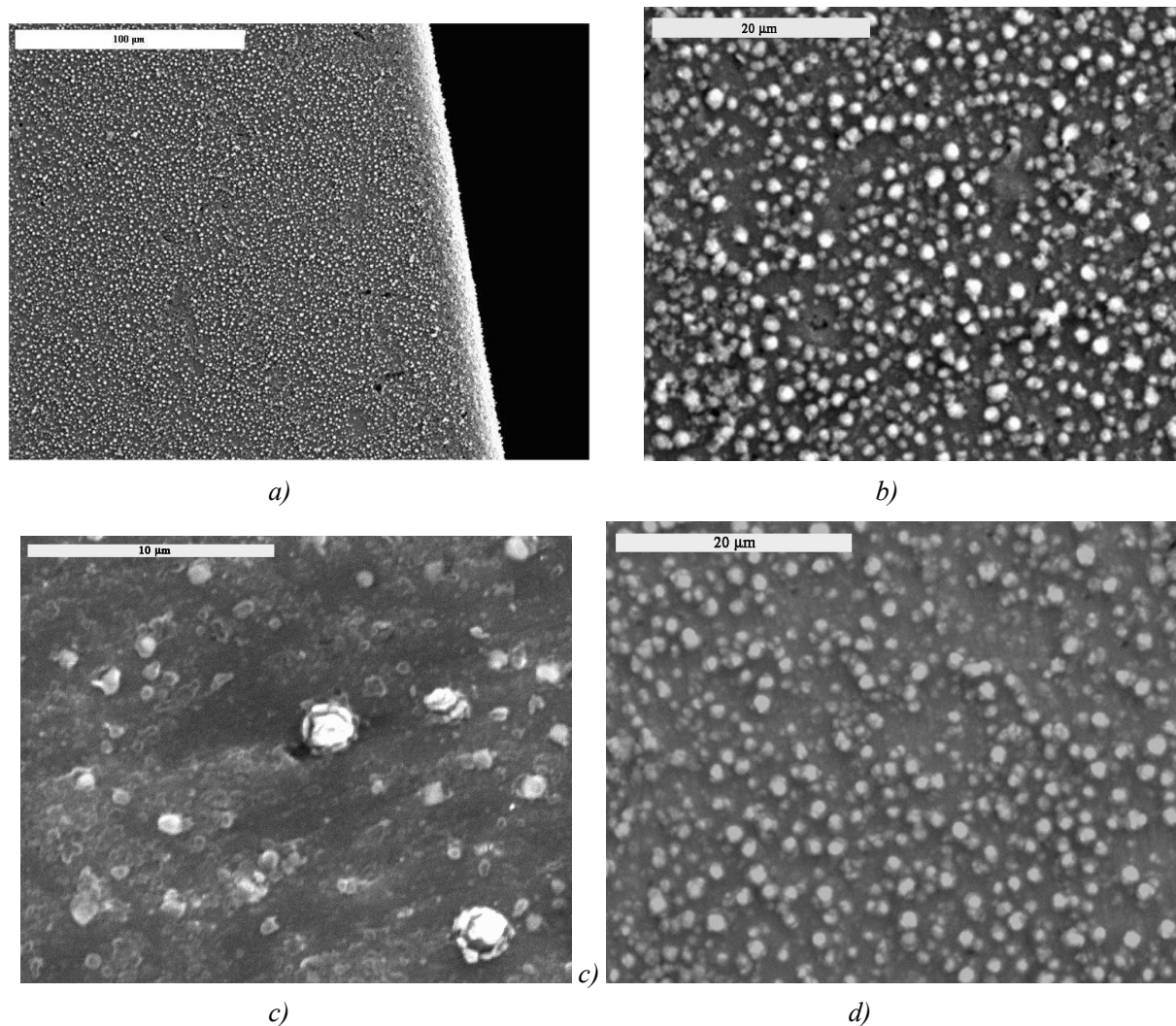
Slika 3 – SEM mikrofotografije površine anodiziranog titana, termički netretiranog, veličina oznake: 100 μm (a), 20 μm (b) i 10 μm (c) i termički tretiranog, veličina oznake: 20 μm (d)
