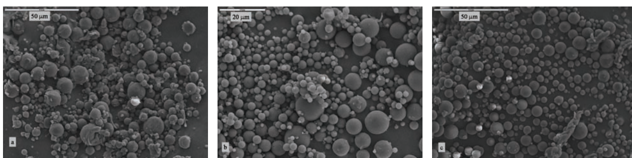
Slika 4. SEM slike mikrosfera dobijenih pri različitim udelima PVA: a) 0,2, b) 0,5 i c) 1,0 mas. %.
