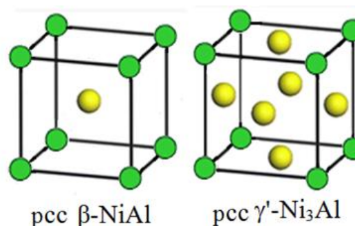
Slika 2. Prostorno centrirana kubna \beta -NiAl i površinski centrirana kubna rešetka \gamma' -Ni 3 Al faza
