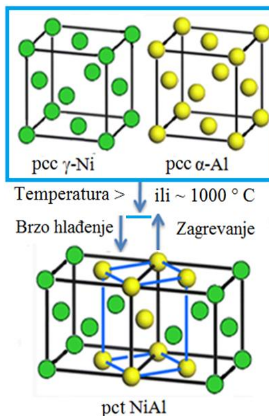
Slika 3. NiAl martenzit sa površinski centriranom tetragonalnom rešetkom
