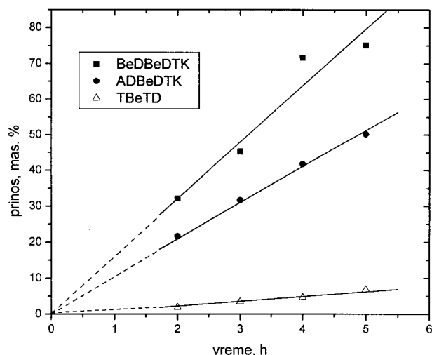
Slika 2. Zavisnost prinosa PMMA od vremena fotohemijske polimerizacije MMA u benzenu inicirane BeDBeDTK –om, ADBeDTK–om i TBeTD–om ( T_p = 25^\circ\text{C} , [In] = 2,0 \text{ mas.}\% , V_{\text{MMA}} = 5,0 \text{ cm}^3 , V_{\text{ben}} = 5,0 \text{ cm}^3 )
