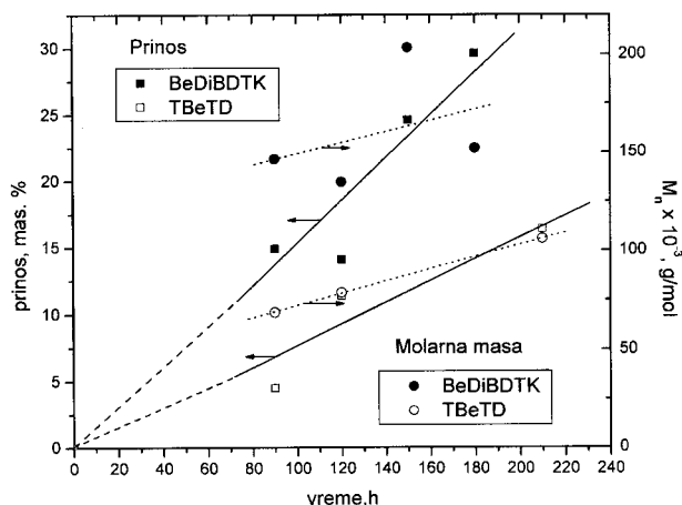
Slika 1. Zavisnost prinosa i M_n od vremena fotohemijške polimerizacije MMA u masi inicirane BeDiBDTK-om i TBeTD-om ( [BeDiBDTK] = 6,78 \times 10^{-3} mol dm -3 ; [TBeTD] = 3,55 \times 10^{-3} mol dm -3 , T_p = 25^\circ\text{C} )
