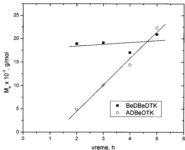
Slika 3. Zavisnost molarne mase PMMA od vremena fotohemijske polimerizacije MMA u benzenu inicirane BeDBeDTK –om i ADBeDTK–om ( T_p = 25^\circ\text{C} , [In] = 2,0 \text{ mas.}\% , V_{\text{MMA}} = 5,0 \text{ cm}^3 , V_{\text{ben}} = 5,0 \text{ cm}^3 )
