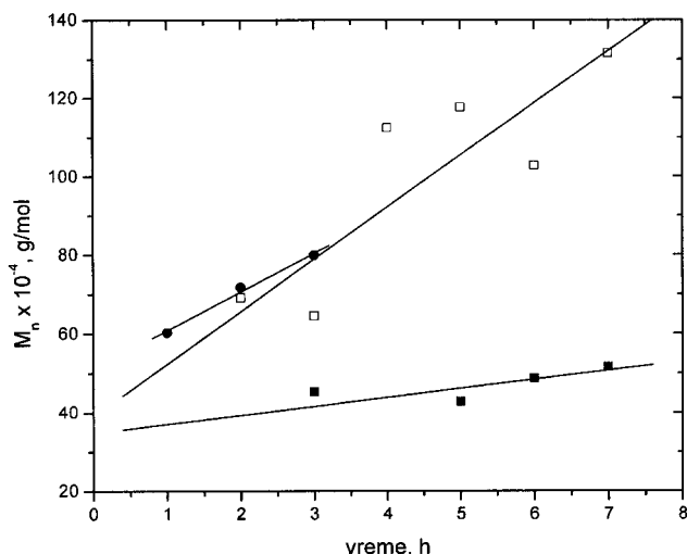
Slika 5. Zavisnost molarne mase PMMA od vremena za termički iniciranu polimerizaciju MMA u: □ – masi, ■ – toluenu i ● – dimetilacetamidu pri temperaturi od 90°C (uslovi polimerizacije su isti kao uz sliku 4)
