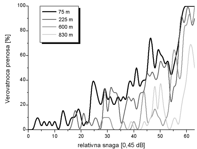
Slika 3. Verovatnoća prenosa paketa u zavisnosti od predajne snage na različitim udaljenostima prijemnika
