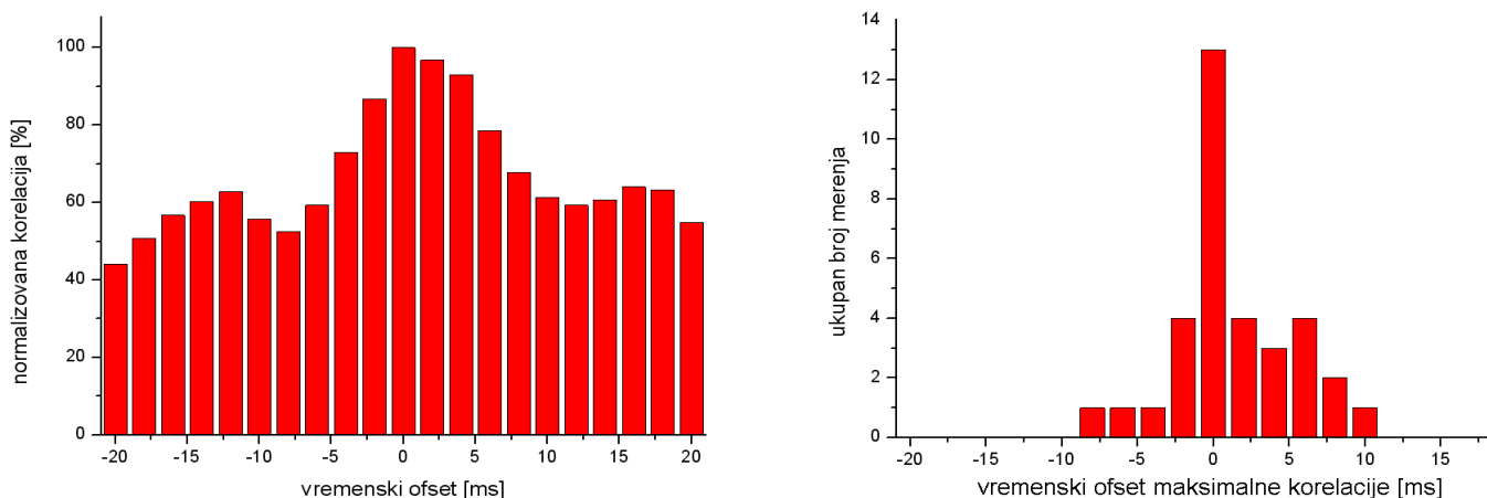
Slika 2. Histogrami kros-korelacije u zavisnosti od vremenskog ofseta snimljenih signala
