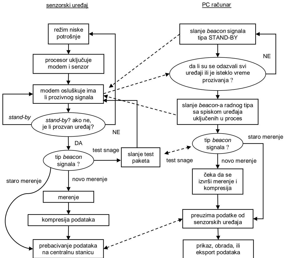
Slika 1 - Algoritam rada sistema
