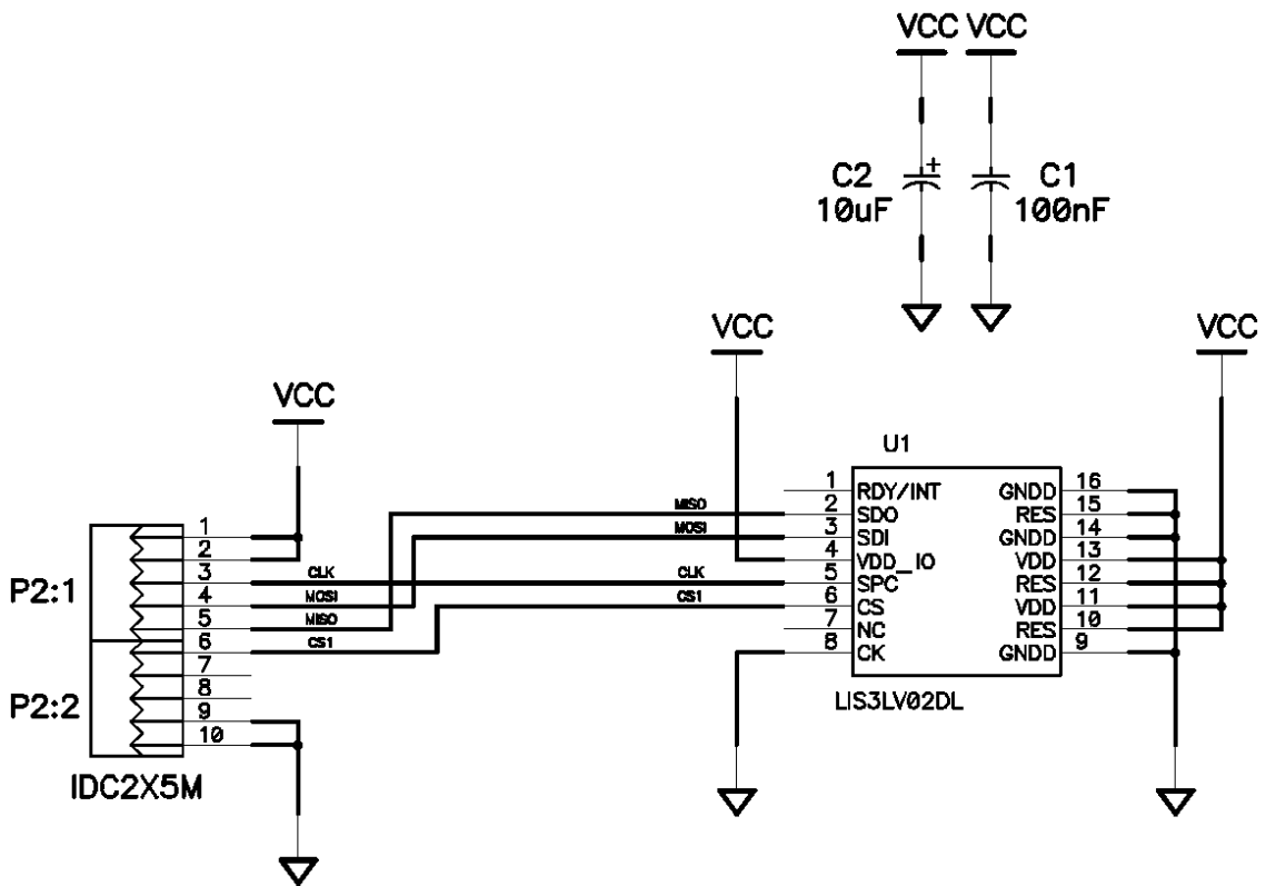
Slika 12.4 Akcelerometar
